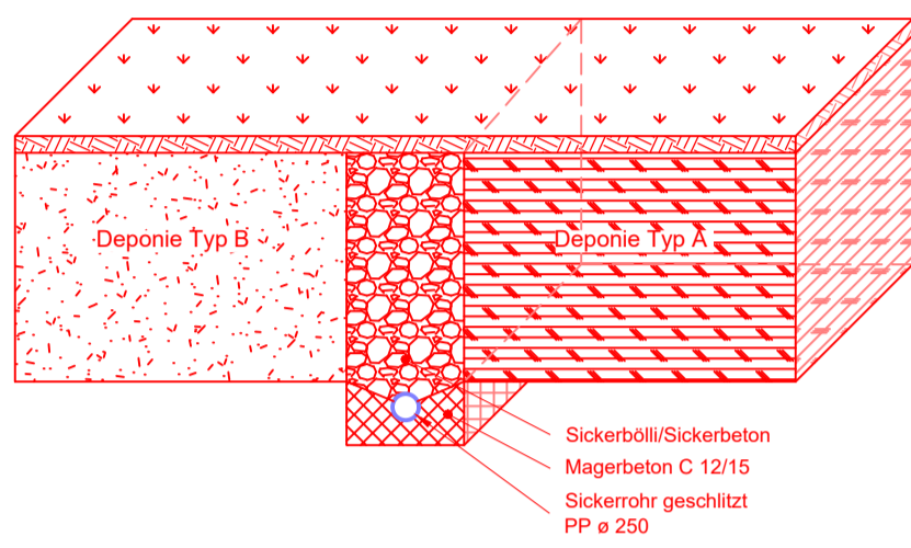
SCHEMASCHNITT SICKERVORHANG 1 : 50
